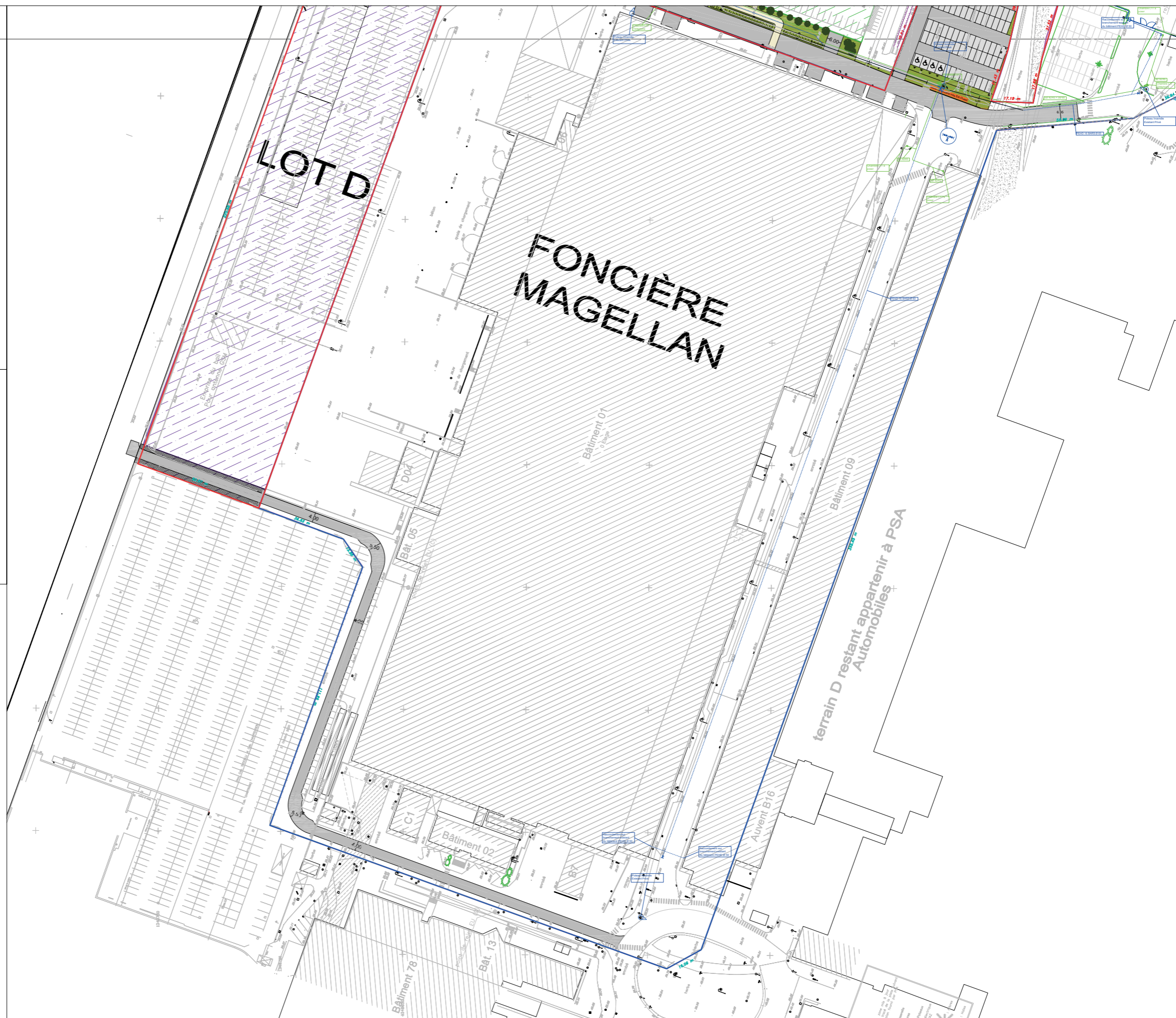
Figure 49 : Plan réseaux AEP - TELECOM - Planche 2
